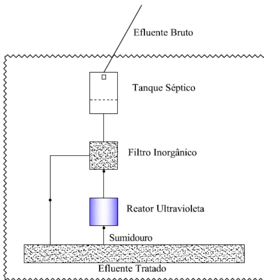
FIGURA 1. Ilustração da unidade de tratamento de esgoto doméstico implantado no parque Zoobotânico da UFRSA, em Mossoró-RN.
