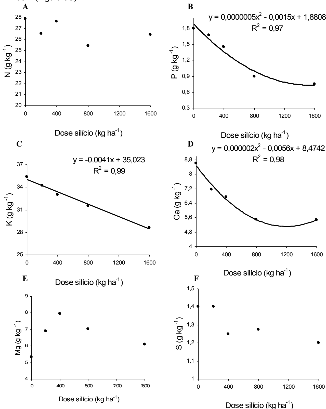
Figura 5. Efeito de doses de escória siderúrgica sobre os teores foliares de N (A), P (B), K (C), Ca (D), Mg (E) e S (F) após o cultivo da brachiaria.
